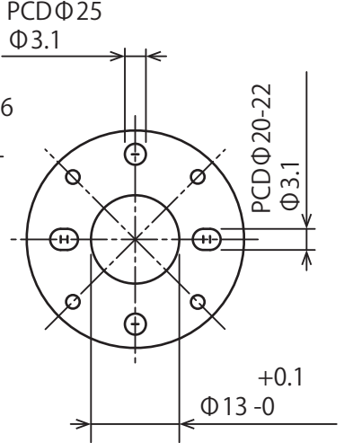
FP仕様フランジ
