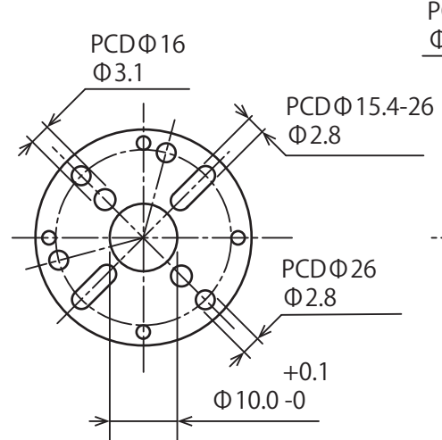
FS仕様フランジ
